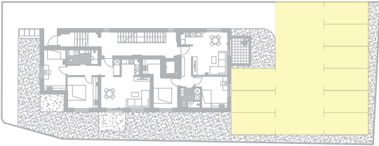
TLOCRT PRIZEMLJA
